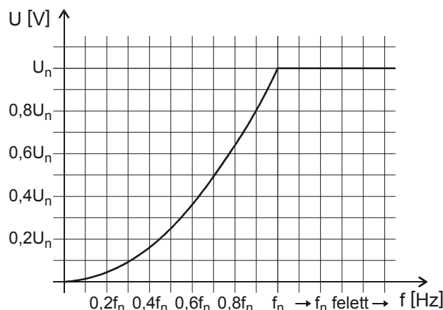
Négyzetes U/f alap-karakterisztika Típus-karakterisztika: normál Négyzetes módosítás: 100% U indító: 0V
