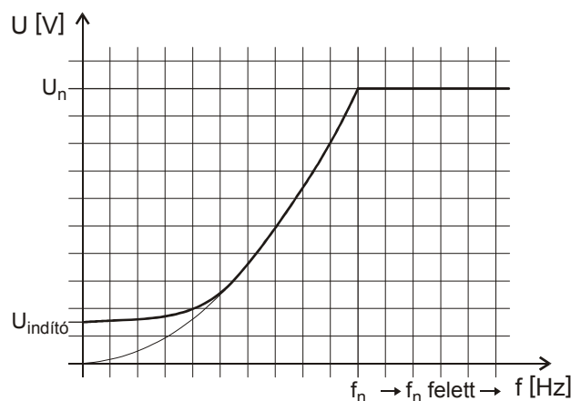
Négyzetes U/f felhasználói-karakterisztika Típus-karakterisztika: normál Négyzetes módosítás: 100% U indító: beállítva
